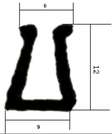
T/7 Guarnizione infissi vetri multi usi
